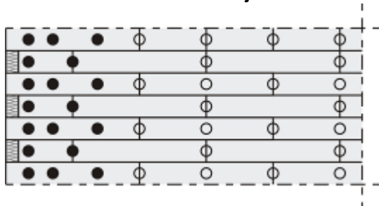
12 hmoždinek/m 2 na nároží objektu
