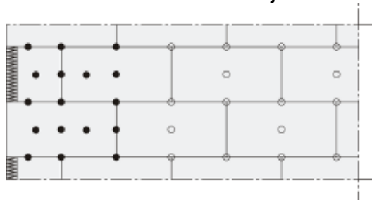
12 hmoždinek /m 2 na nároží objektu
