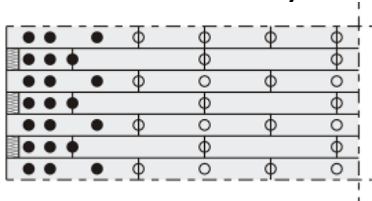
14 hmoždinek /m 2 na nároží objektu
