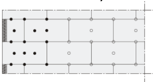
10 hmoždinek/m 2 na nároží objektu
